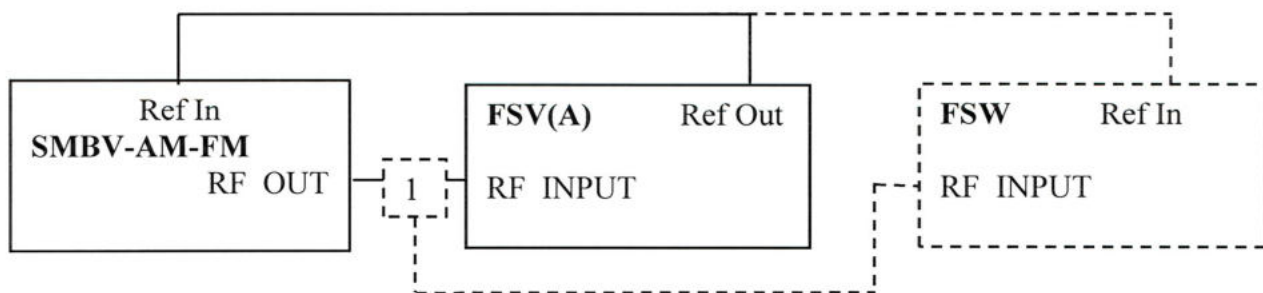
1 – делитель мощности СВЧ
