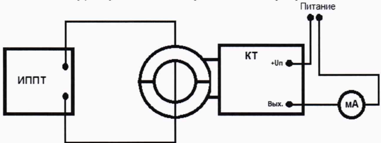
Рисунок 3 – Схема измерений при определении погрешности преобразования силы постоянного тока для клещей токоизмерительных КТ-***-У-4/20-Д54
