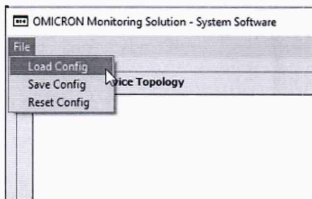
Рисунок 15 – Загрузка конфигурации
