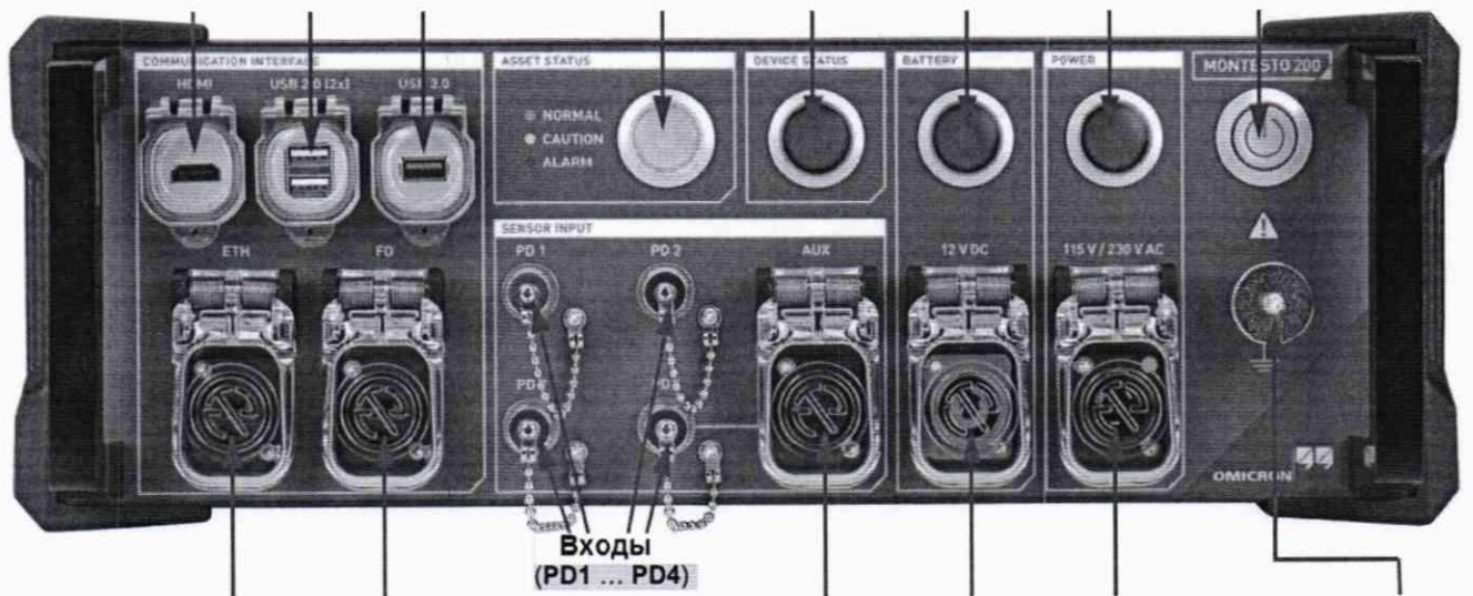
Рисунок 33 – Передняя панель системы MONTESTO 200
