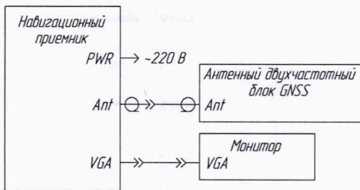
Рисунок 1 — Схема подключения CM-ГЛОНАСС для проверки работоспособности
