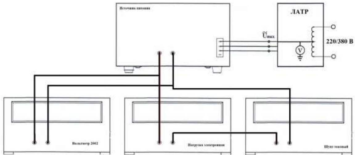
Рисунок 7 – Структурная схема соединения приборов для определения абсолютной погрешности измерения мощности переменного тока
