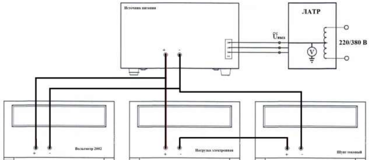
Рисунок 8 – Структурная схема соединения приборов для определения абсолютной погрешности воспроизведения мощности постоянного тока
