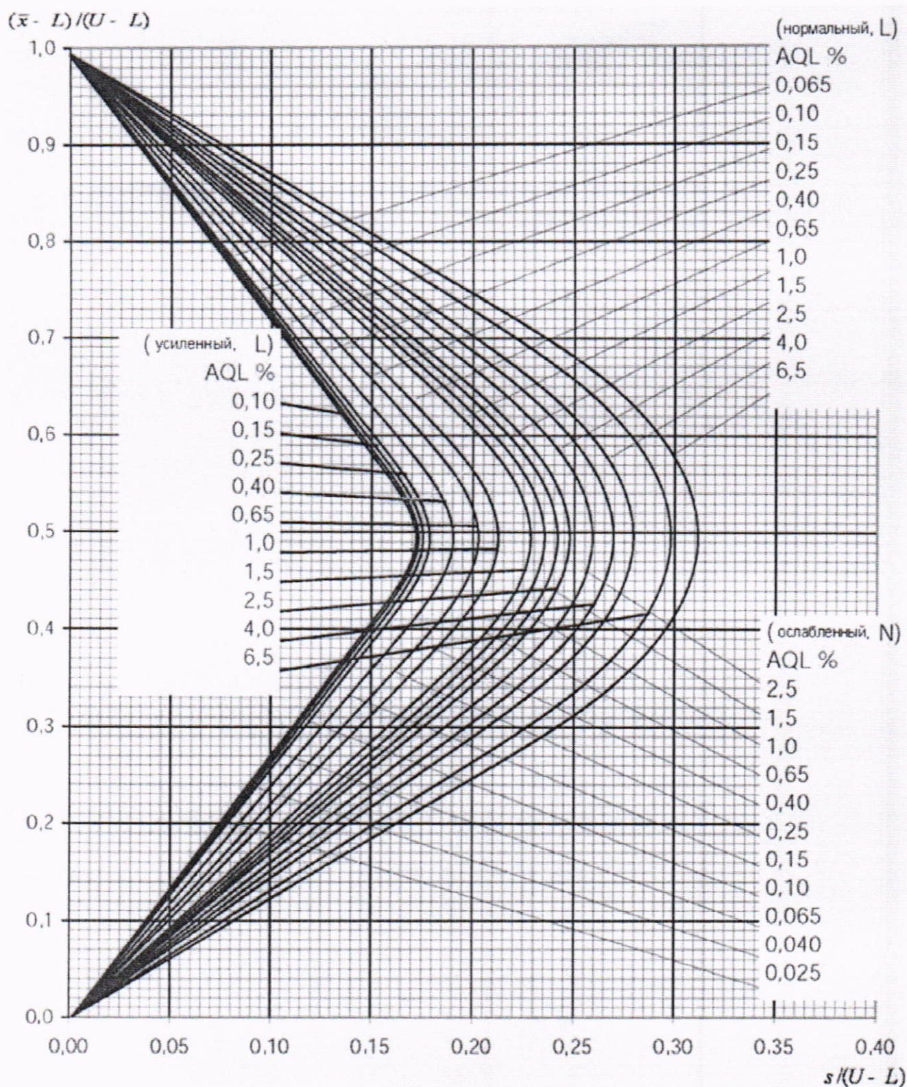
Рисунок Г.8 – График s-L. Приемочные кривые для объединенного контроля с двумя границами поля допуска для кода объема выборки L при нормальном и усиленном контроле и для кода объема выборки N при ослабленном контроле
