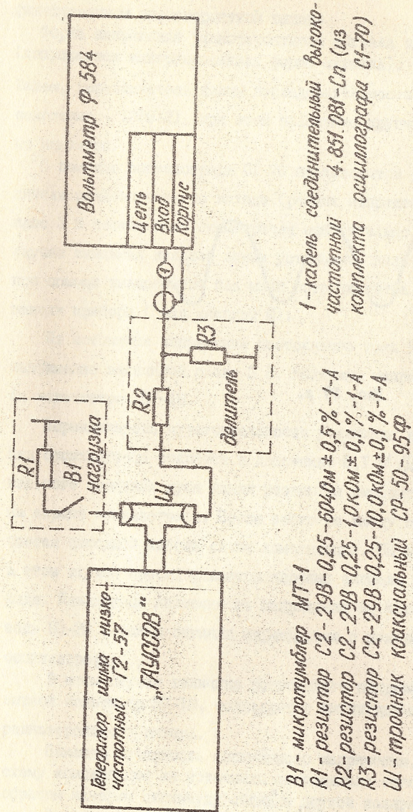
Рис. 27. Схема электрическая соединений для проверки эффективного значения напряжения и выходного сопротивления на фиксированном гауссовом выходе
