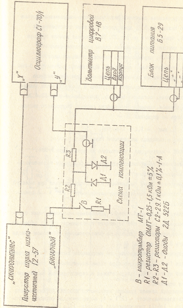
Рис. 26 б. Схема электрическая соединений для проверки напряжения сигнала на фиксированном бинарном выходе при периоде тактовой частоты - 1 \mu S (Микроимпульс В отключен)
