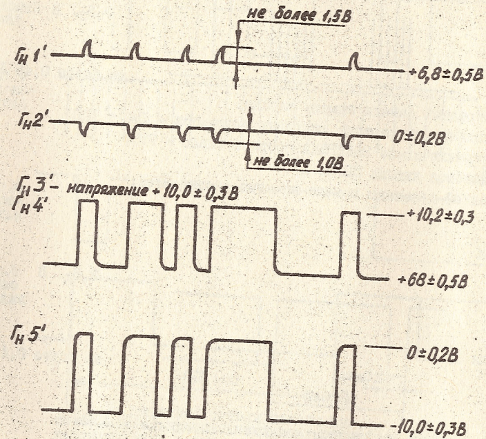
Осциллограммы напряжений и уровни напряжений на контрольных гнездах платы 5.002.067
