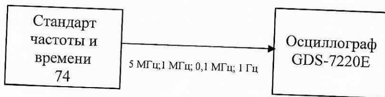
Рисунок 3 - Схема измерений частот выходных импульсных сигналов
