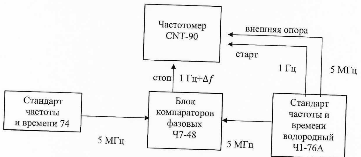
Рисунок 4 – Схема измерений значений относительной разности частот
