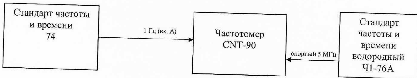
Рисунок 1 - Определение периода импульсного сигнала 1 Гц
