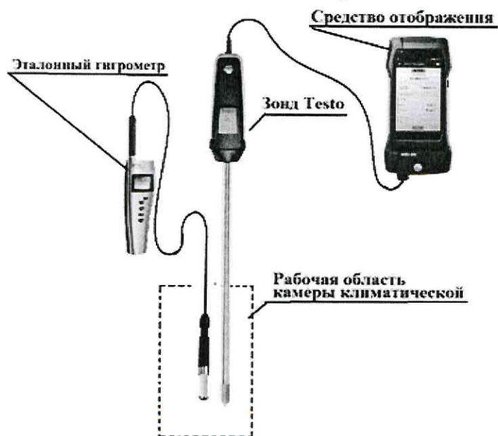
Рисунок 3 – Схема определения абсолютной погрешности измерений относительной влажности методом непосредственного сличения
