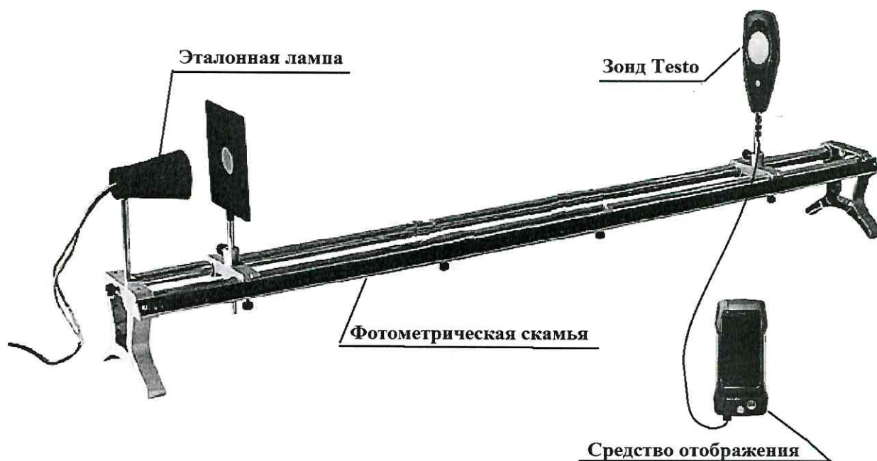
Рисунок 8 – Схема установки зонда Testo на фотометрической скамье
