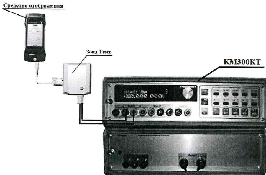
Рисунок 9 – Схема подключения зонда Testo к компаратору-калибратору универсальному KM300KT при определении абсолютной погрешности измерений напряжения постоянного тока
