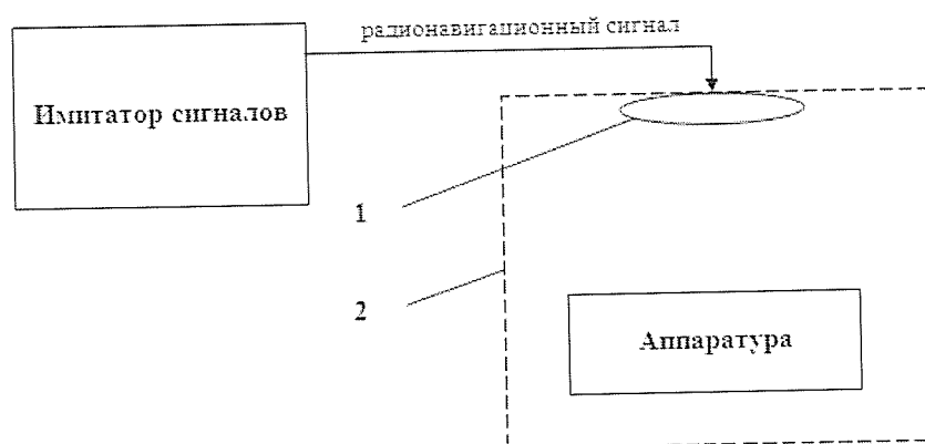
Рисунок 1 – Схема измерений
