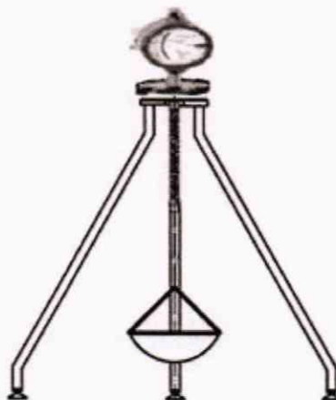
Рисунок 1 – Монтаж уровнера
