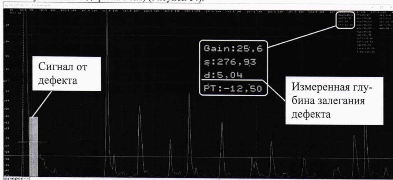
Рисунок 14 – А-развёртка при измерении глубины залегания отражателя
