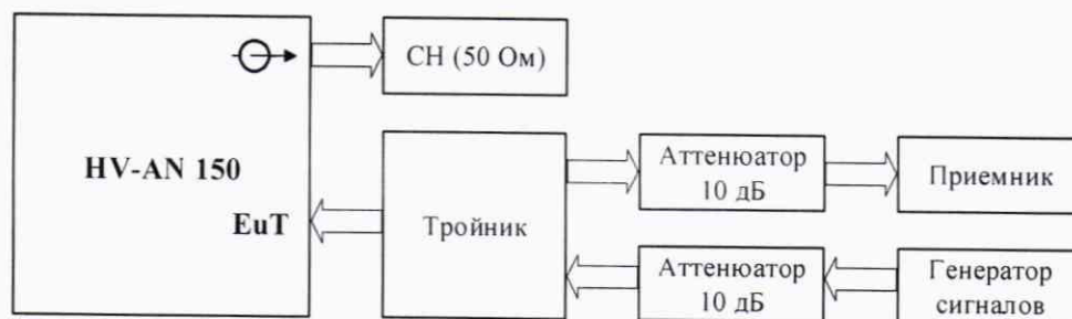
Рисунок 1 - Схема калибровки выходного уровня генератора сигналов
