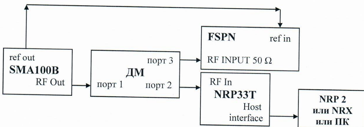
Рисунок 2 – Структурная схема соединения СИ для определения абсолютной погрешности измерения уровня мощности входного сигнала, в диапазоне частот
