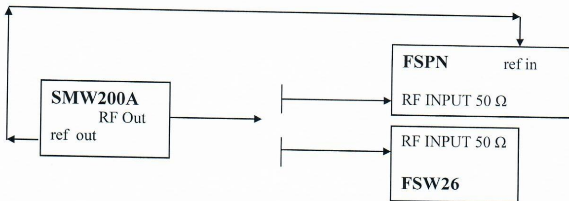
Рисунок 3 – Структурная схема соединения СИ для определения абсолютной погрешности измерения фазового шума входного сигнала
