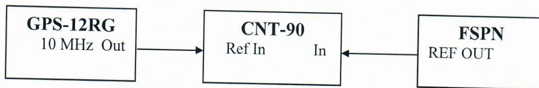
Рисунок 1 – Структурная схема соединения СИ для определения относительной погрешности частоты опорного генератора
