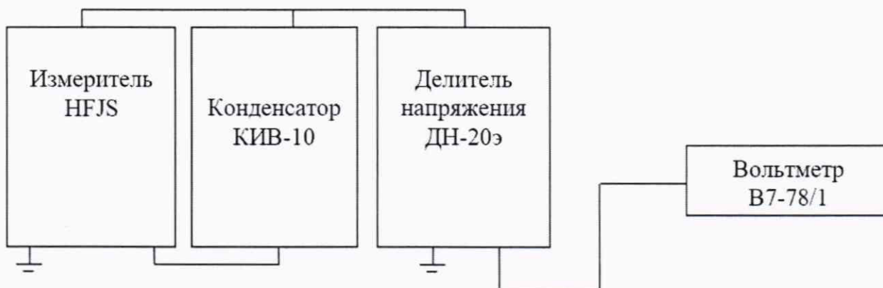
Рисунок 2 – Схема проверки абсолютной погрешности воспроизведений напряжения и частоты переменного тока
