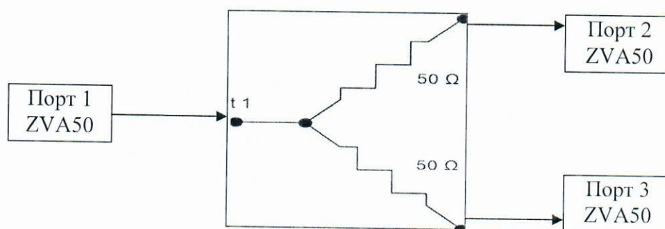
Рисунок 4 – Структурная схема соединения СИ для определения коэффициента передачи резистивного делителя мощности
