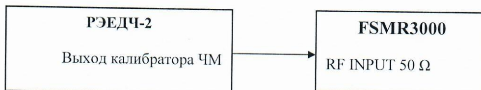
Рисунок 7 – Структурная схема соединения СИ для определения абсолютной погрешности измерений девиации частоты на несущих частотах 5 МГц и 50 МГц
