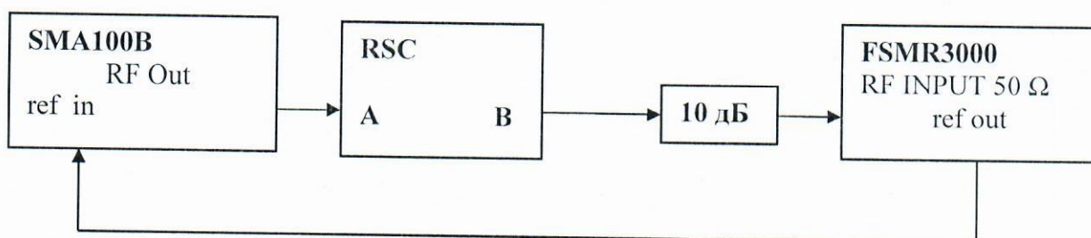
Рисунок 9 – Структурная схема соединения СИ для определения абсолютной погрешности измерений уровня мощности входного сигнала из-за переключения ослабления аттенюатора СВЧ
