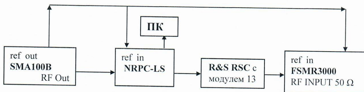
Рисунок 3 – Структурная схема соединения СИ для определения абсолютной погрешности измерений ослабления в диапазоне частот
