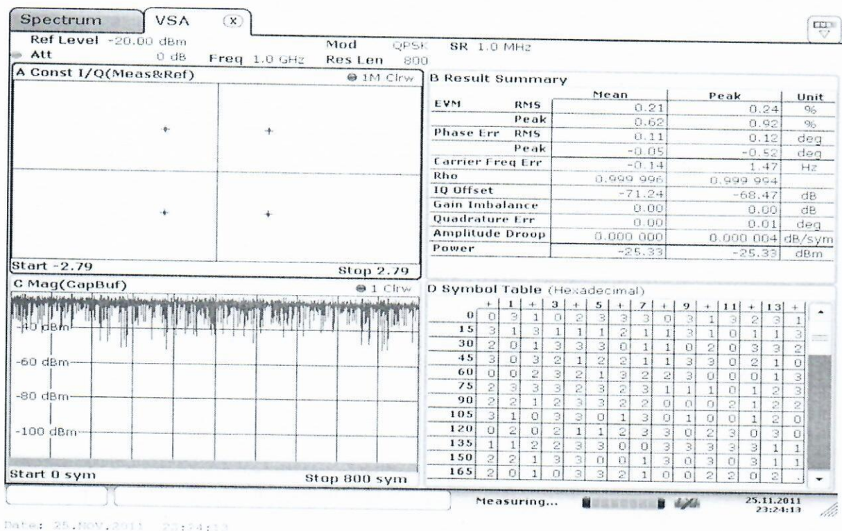
Рисунок 13 – меню приемника в режиме измерений модуляции типа QPSK
