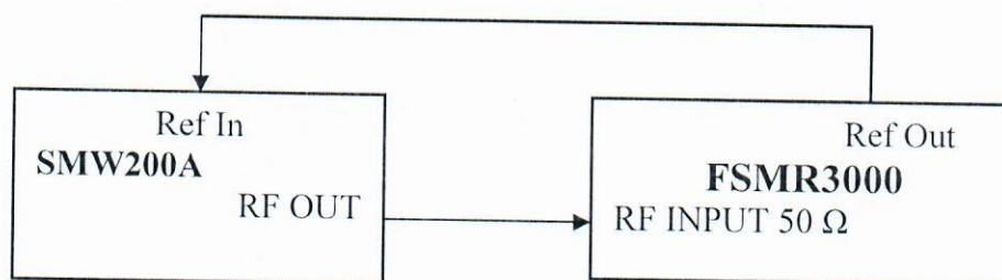
Рисунок 12 – Структурная схема соединения СИ для определения остаточного среднеквадратического значения векторной ошибки модуляции для модуляции QPSK
