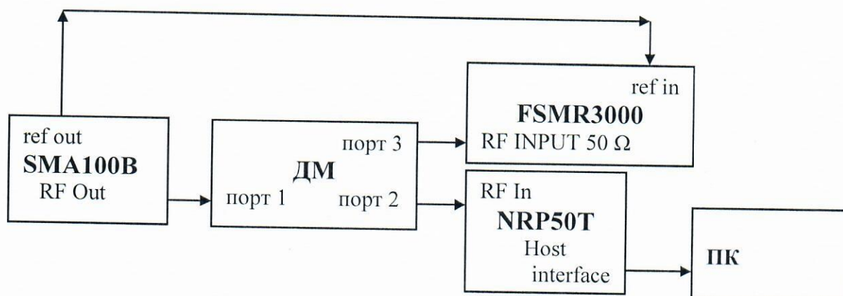
Рисунок 5 – Структурная схема соединения СИ для определения абсолютной погрешности измерений уровня мощности в диапазоне частот
