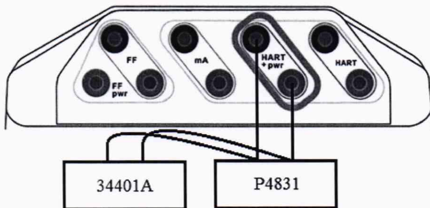
Рисунок 7 – Схема подключения средств поверки к разъему коммутатора HART+pwr при определении погрешности воспроизведений силы постоянного тока
