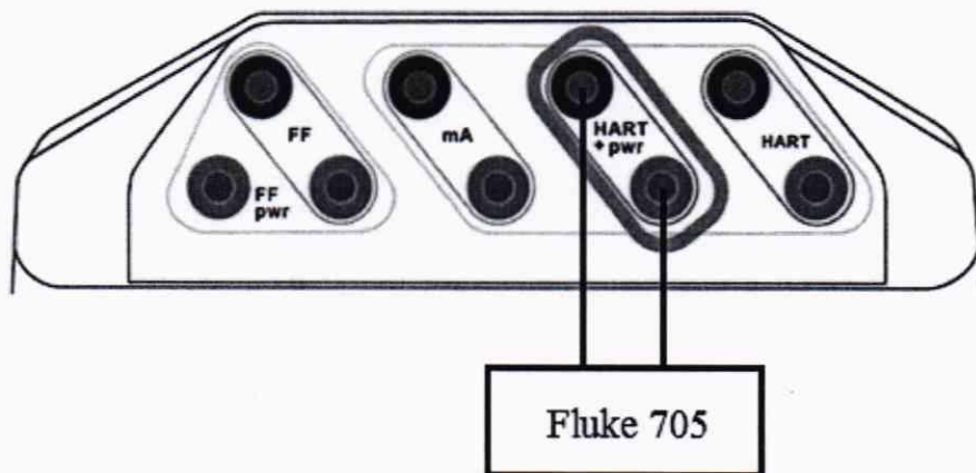
Рисунок 3 – Схема подключения средств поверки к разъему коммуникатора HART+pwr при определении погрешности измерений силы постоянного тока (способ 1)
