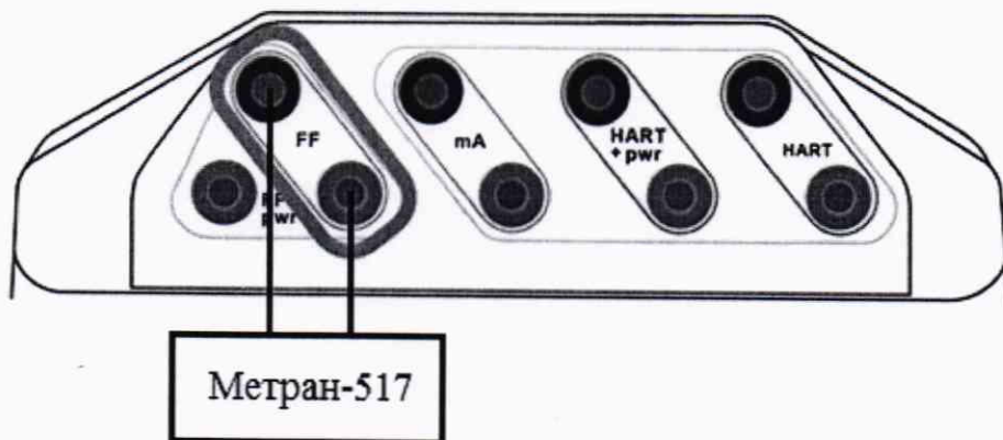
Рисунок 2 – Схема подключения средств поверки к разъему коммуникатора FF при определении погрешности измерений постоянного напряжения
