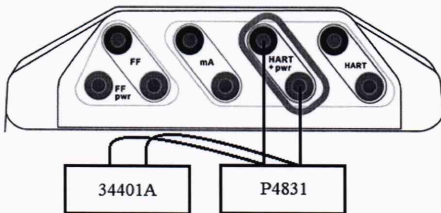
Рисунок 4 – Схема подключения средств поверки к разъему коммуникатора HART+pwr при определении погрешности измерений силы постоянного тока (способ 2)
