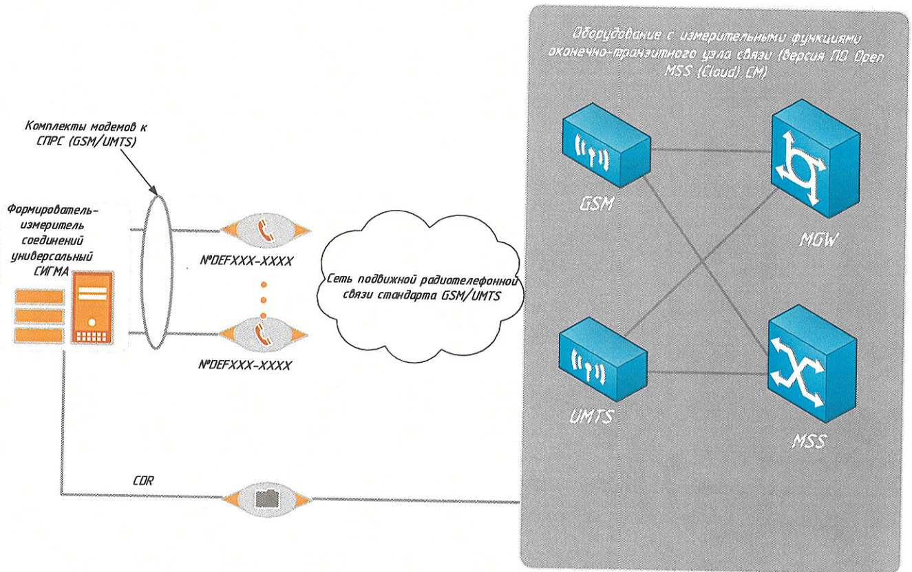
Рисунок 1 – Схема поверки СИПД
