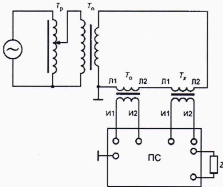
Рисунок 2 - Схема поверки с использованием рабочего эталона и прибора сравнения (компаратора вторичных токов)
