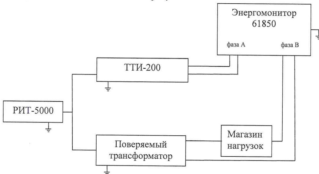
Рисунок 1 – Схема определения токовых и угловых погрешностей
