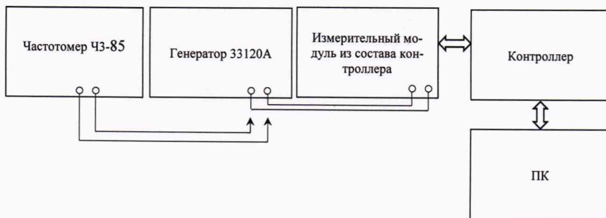
Рисунок 4 – Схема подключения при преобразовании количества импульсных сигналов
