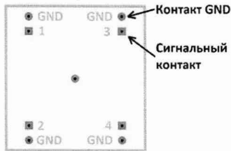
Рисунок 13 – Контакты для калибровки устройства TSKY.418133.416
