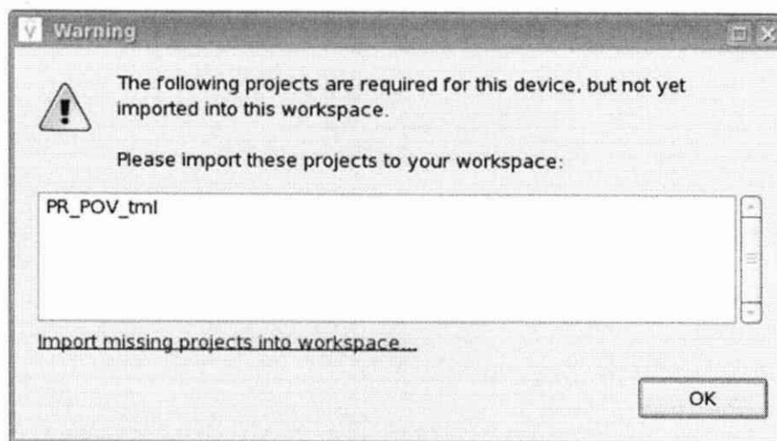
Рисунок 4 – Окно Warning
