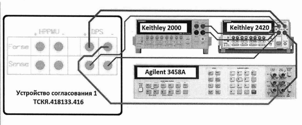
Рисунок 24 – Схема определения погрешности воспроизведения (измерения) напряжения и измерения (воспроизведения) силы тока источником питания DCS DPS128
