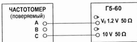
Рисунок 8.1 - Схема подключения приборов при измерении интервалов времени
