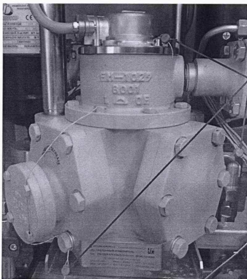
Р и с у н о к Б . 1 – Схема пломбировки измерителя объема поршневого типа FM-1029
