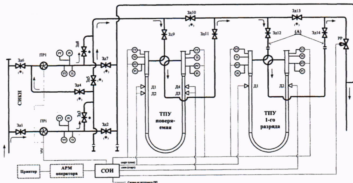
Рисунок 1 Принципиальная схема соединений поверяемой ТПУ и средств поверки при использовании РР, установленного на СИКН, в качестве компаратора. РР1 – контрольно-резервный РР (при наличии в составе СИКН); РРi – рабочий РР, установленный на i-ой ИЛ; РТ – измерительный преобразователь избыточного давления; РI – манометр; ТТ – датчик температуры; Д1...Д4 – детекторы ТПУ; СОИ; Зд1...Зд14 – задвижки (шаровые краны); РР – регулятор расхода.
