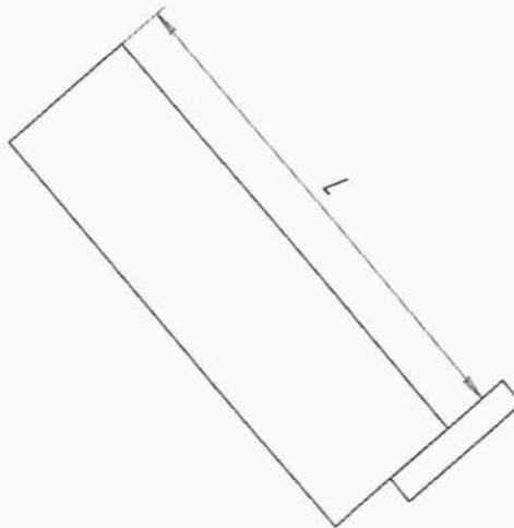
Рисунок 1 – Расположение концевых мер и измеряемый параметр
