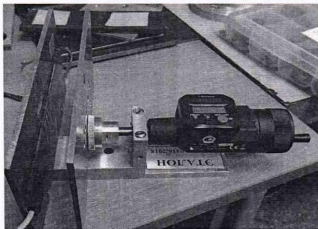
Рисунок 1 – Юстировочное устройство.
