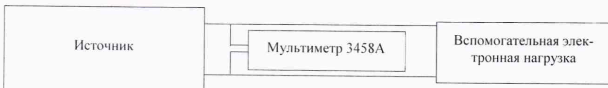
Рисунок 1 – Структурная схема определения абсолютной погрешности воспроизведений/измерений напряжения постоянного тока
