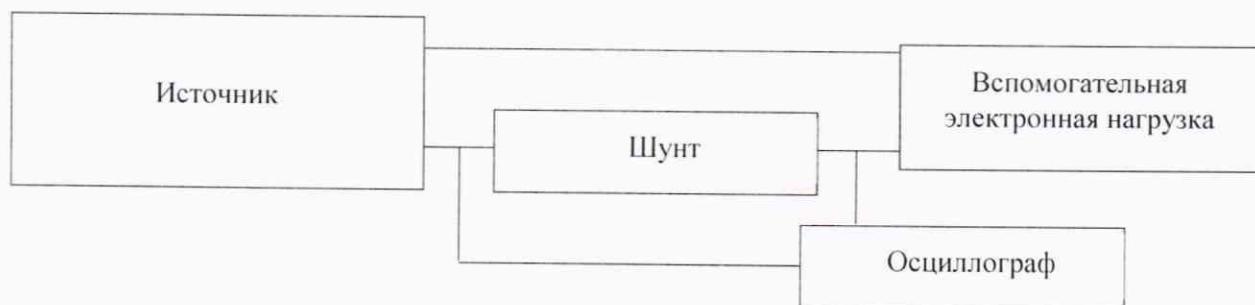
Рисунок 7 - Структурная схема определения уровня пульсаций выходного сигнала силы постоянного тока в режиме стабилизации силы постоянного тока
