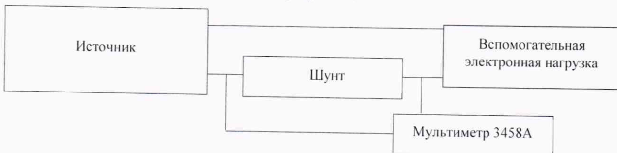
Рисунок 2 – Структурная схема определения абсолютной погрешности воспроизведений/измерений силы постоянного тока
