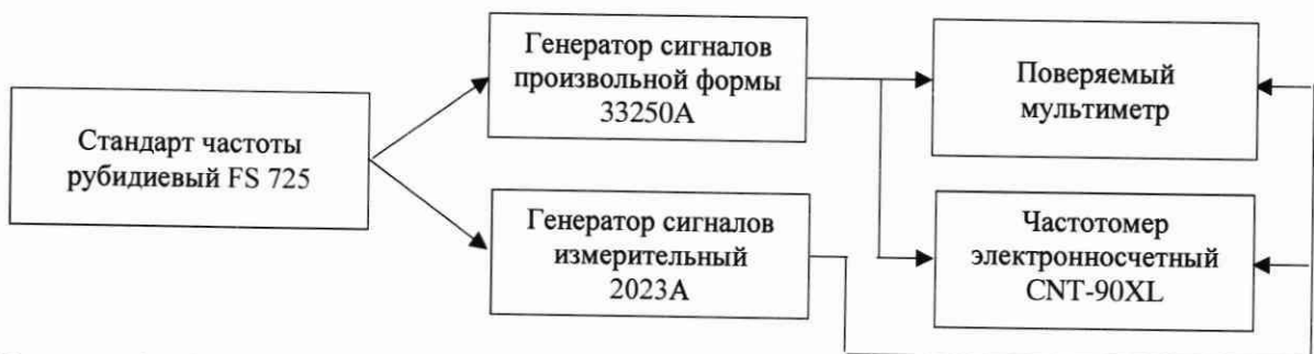
Рисунок 8 - Схема соединения приборов при поверке мультиметра в режиме измерений частоты
