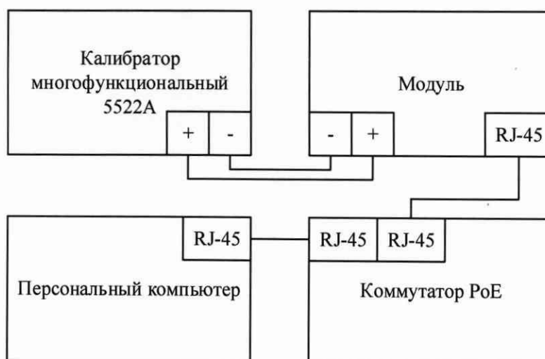
Рисунок 1 – схема определения приведенной (к верхнему пределу измерений) погрешности измерений силы постоянного тока
