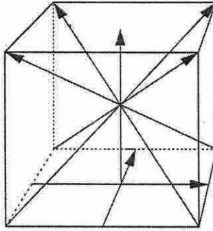
Рисунок 1 - Типичные положения, в которых производят измерения в пределах объема КИМ
