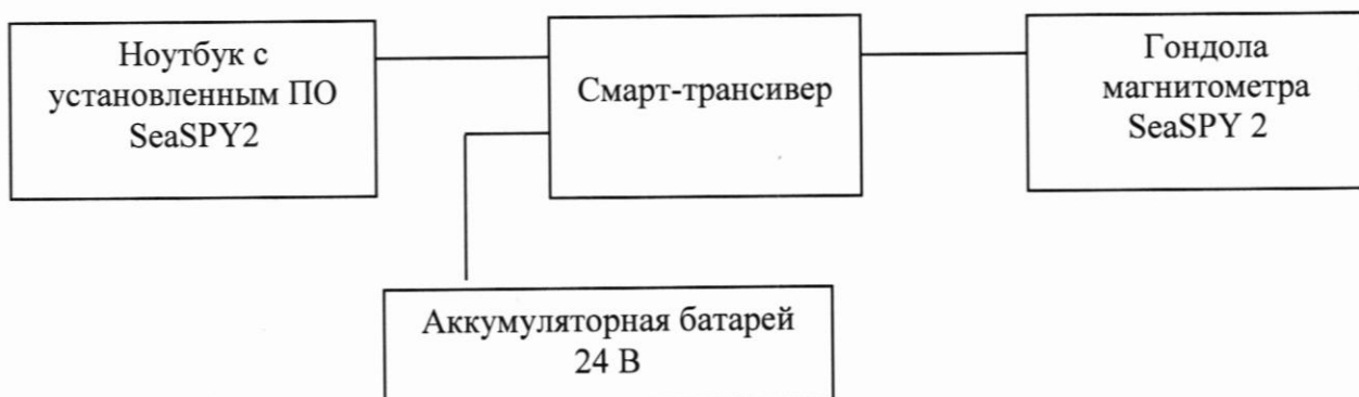
Рисунок 1 - Схема подключения
