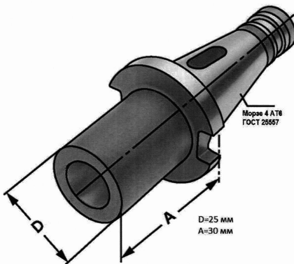
Рисунок 1 – Эскиз переходника
