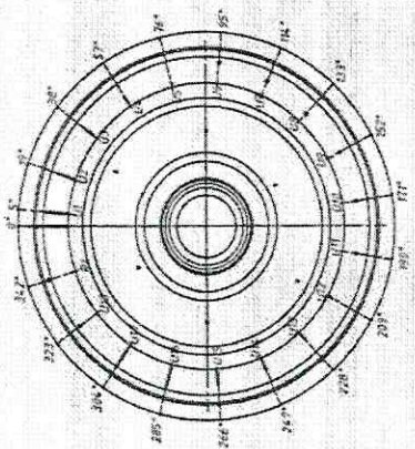
Искусственные отражатели на ободке
