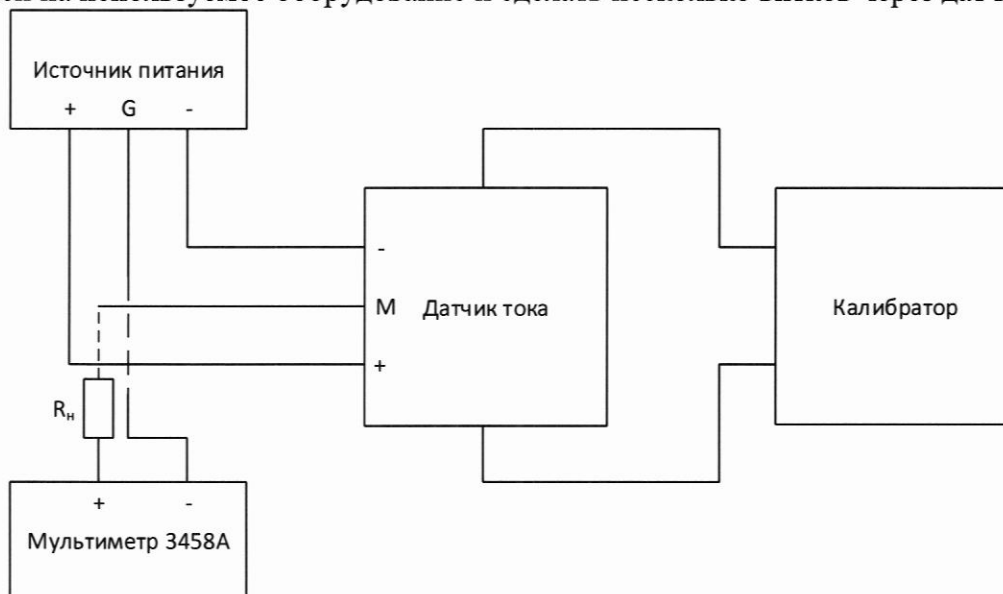
Рисунок 1 – Схема подключения
