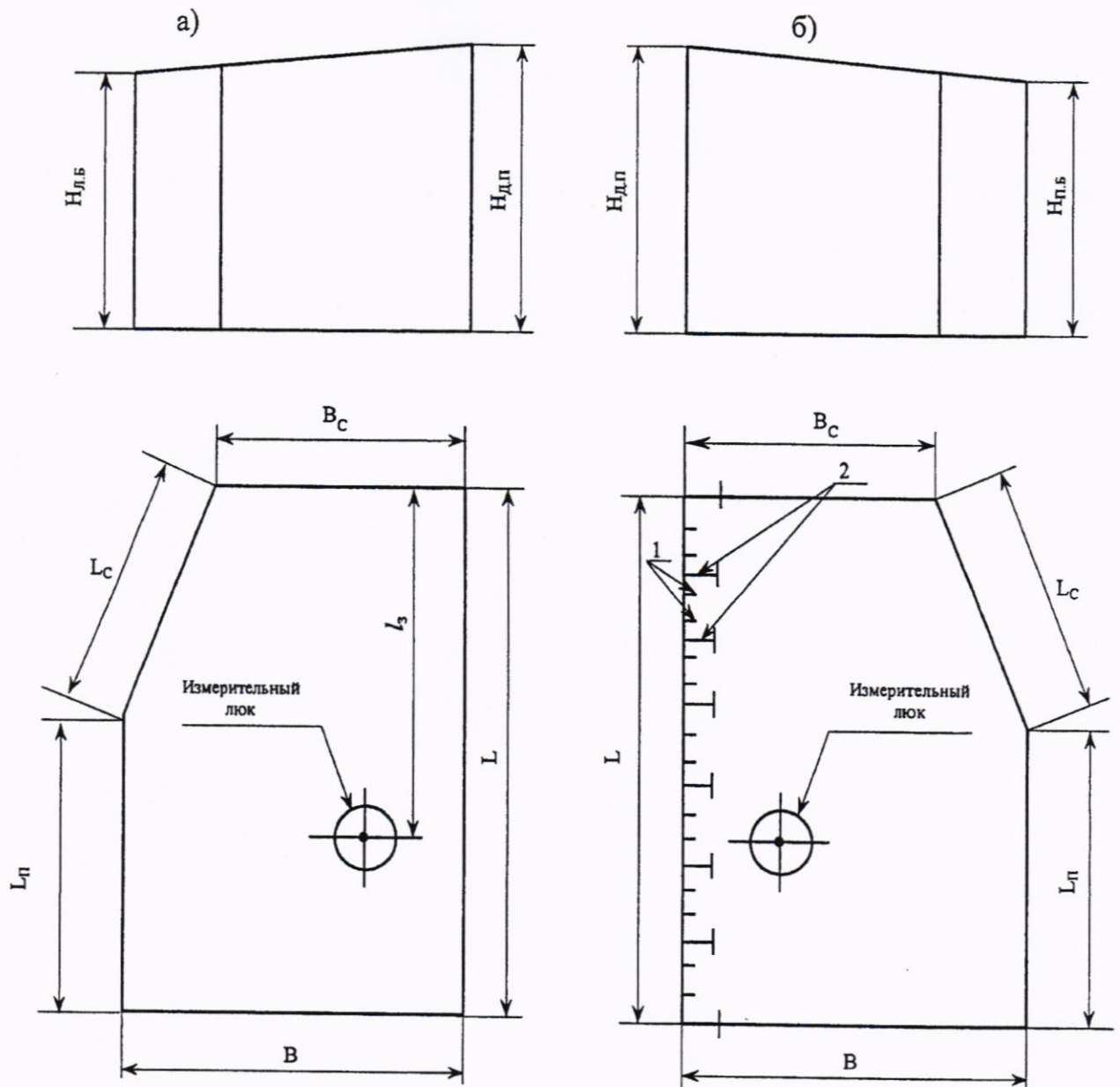
а - танк левого борта; б - танк правого борта; 1 - шпации; 2 - рамные шпангоуты; H_{л.б.} - высота танка по левому борту; H_{п.б.} - высота танка по правому борту; H_{д.п.} - высота танка по диаметральной плоскости; L - общая длина танка; L_{п.} - длина прямоугольной части; В - ширина танка; B_{с.} - ширина в скошенной части; L_{с.} - длина скоса
