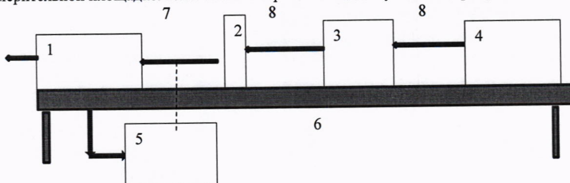
Рисунок 1 Схема определения коэффициента коррекции (калибровки)
