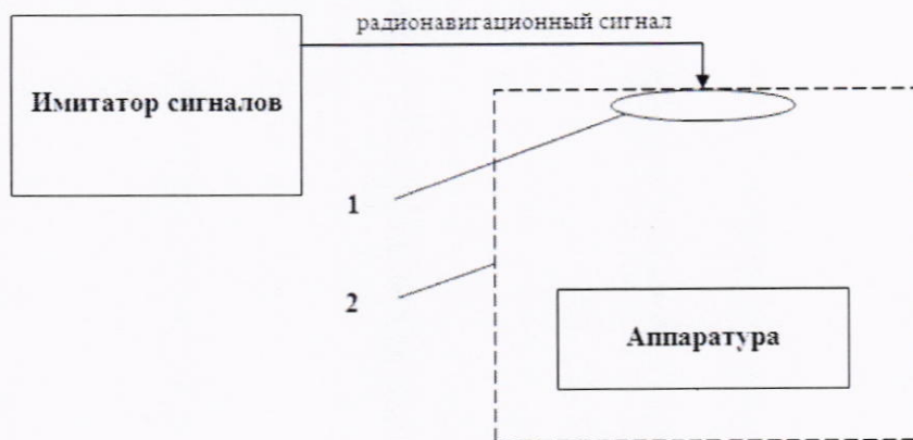
Рисунок 1 – Схема измерений
