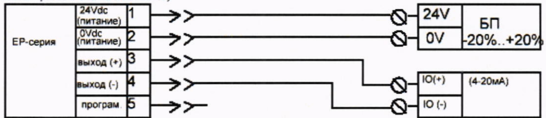
Преобразователь линейного перемещения EP серии (0050M - разъем M12 на 5 контактов)
