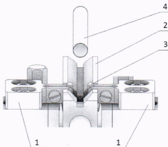
Рисунок 2 – Схема установки мер установочных MarGage 426
