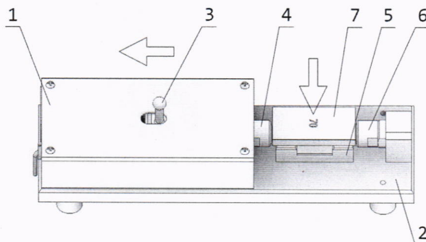
Рисунок 3 – Станция измерительная с индуктивным преобразователем модели БВ-7703.40
