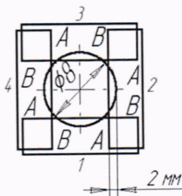
Р и с у н о к 9.3 – Определение отклонения от параллельности плоских измерительных поверхностей
