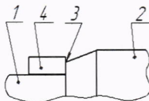
Р и с у н о к 9 . 1 – Определение расстояния от стебля до измерительной кромки барабана у продольного штриха стебля
