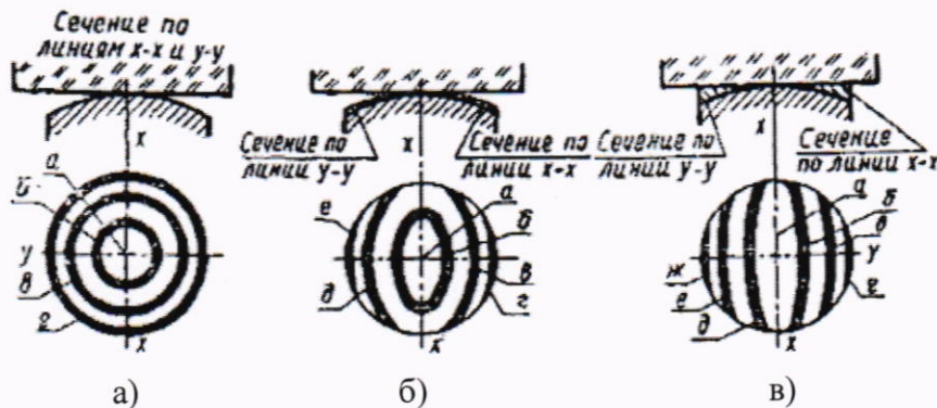
Р и с у н о к 9.2 – Увеличенное изображение картины интерференционных полос (колец) при различных формах отклонений от плоскостности измерительной поверхности микрометра
