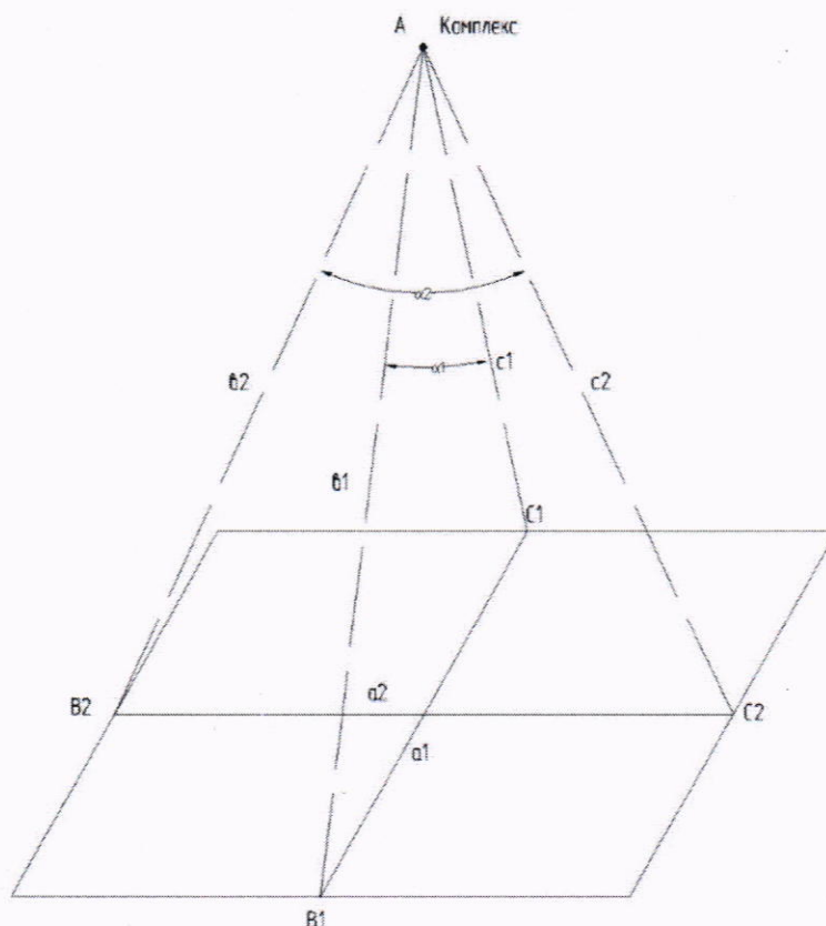
Рисунок 1 – Схема фоторегистрации кадра
