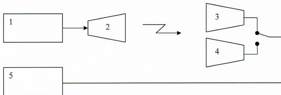
Рисунок 1 Схема измерений
