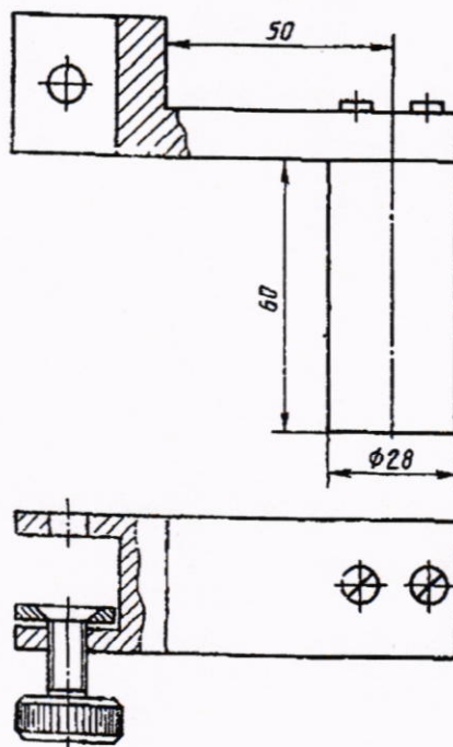
Рисунок Б.1 – Кронштейн
