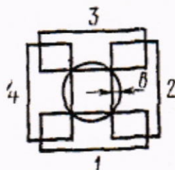
Рисунок 4 – Определение отклонения от параллельности измерительных поверхностей с диапазоном измерений свыше 100 мм
