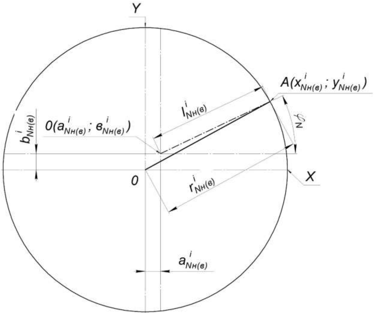
Рисунок Д.2 – Параметры измерений радиуса r_{NH(B)}^i i -го пояса при j -ом измерении в нижнем (верхнем) сечении
