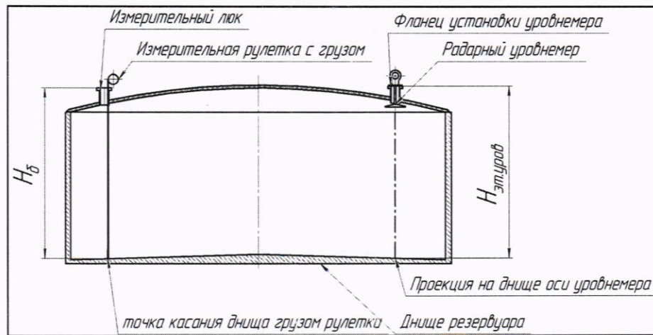
Рисунок А.1 – Схема измерения базовой высоты резервуара и эталонного расстояния урбнмера
