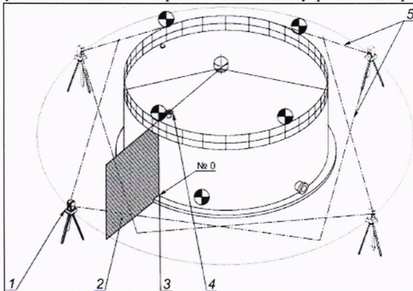
Рисунок А.2 – Схема сканирования методом внутренних измерений
