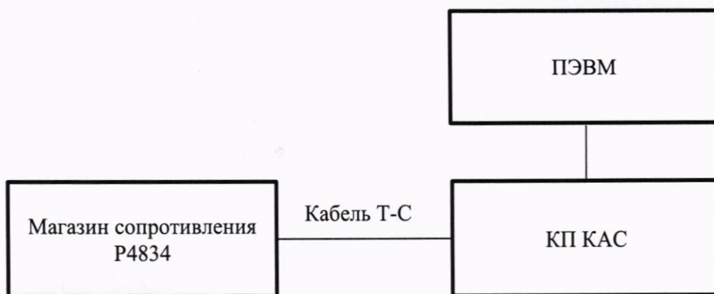
Рисунок 10.3 – Схема подключения
