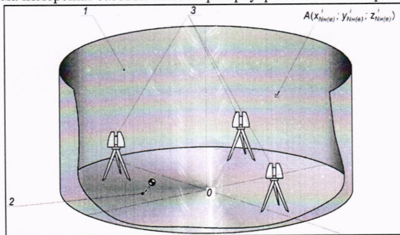
Рисунок А.1 – Схема измерения базовой высоты резервуара и эталонного расстояния уровнера
