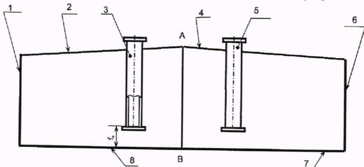
1, 6 – боковые переборки; 2, 4 – палуба судна; 3, 5 – измерительные трубы; 7, 8 – днища танков f_{л} – высота точки касания дна измерительной трубы грузом рулетки; AB – диаметральной плоскости судна
